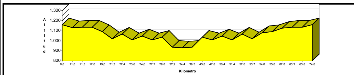
PERFIL ALTIMETRICO
